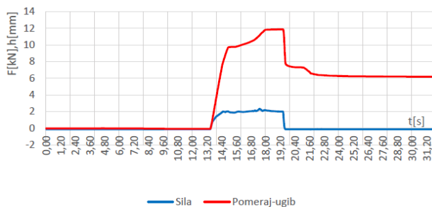
Ispitivanje nosivosti Plafonskog nosača 30x50x30mm proizvođača ITS Kovačević Inđija
