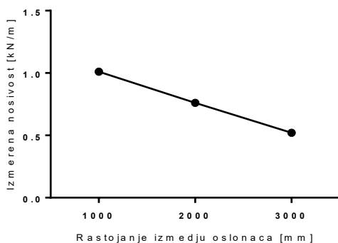
Tip PNK 600/50
