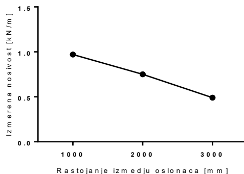
Tip PNK 400/50
