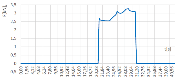
Ispitivanje nosivosti TR nosača proizvođača ITS Kovačević Indija
