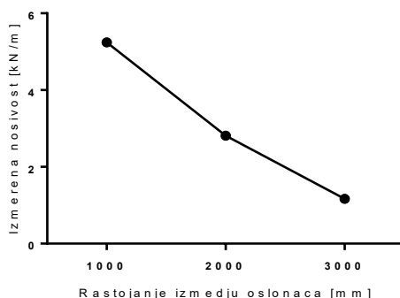
Tip LNK 400/110
