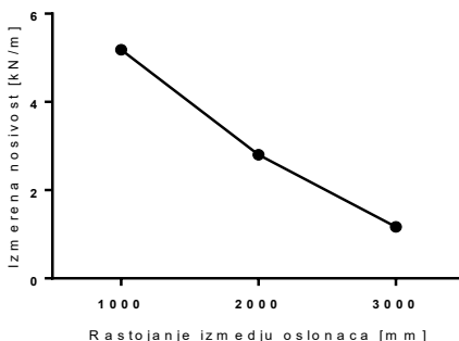
Tip LNK 500/110
