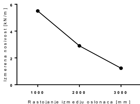
Tip LNK 100/110
